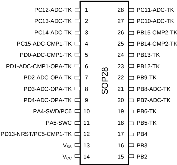
图 3-5 SOP28 Pinout 5 PY32T090G5xS7 (Top view)
